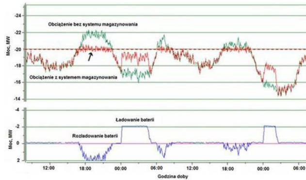
Rys. 9. Praca programowa zasobnika dla potrzeb bilansowania technicznego
