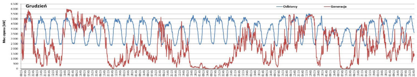
Rys. 8. Zmienność generacji i zapotrzebowania w grudniu (kolorem niebieskim oznaczono zapotrzebowanie, czerwonym generację)
