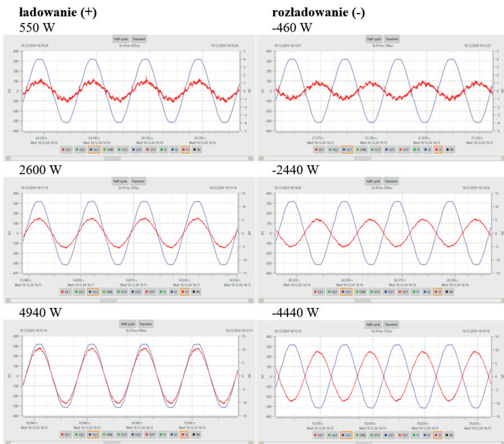
Rys. 21. Przebiegi wartości chwilowych napięć i prądów odpowiadające poziomom ładowania i rozładowania z Rys. 20
