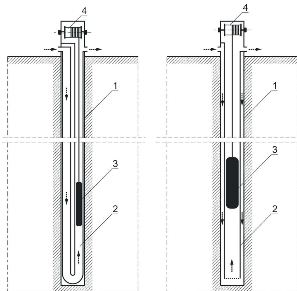
Rys. 23. Otworowy wymiennik ciepła z opcją grawitacyjnego magazynowania energii: 1 – otwór wiertniczy, 2 – rury cyrkulacyjne nośnika ciepła, 3 – obciążnik, 4 – wciągarka
