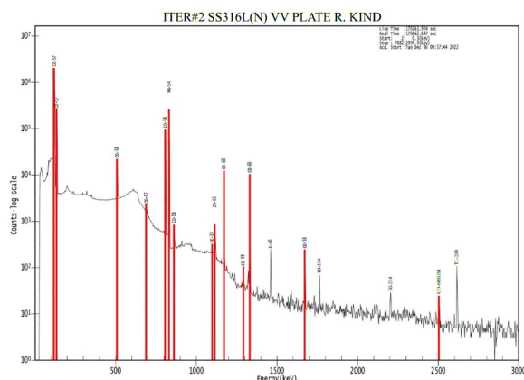
Rys. 3. Widmo promieniowania gamma zarejestrowane dla próbek wykonanej ze stali SS316L(N) zaaktywowanej w trakcie kampanii DTE2 i TT na tokamaku JET
