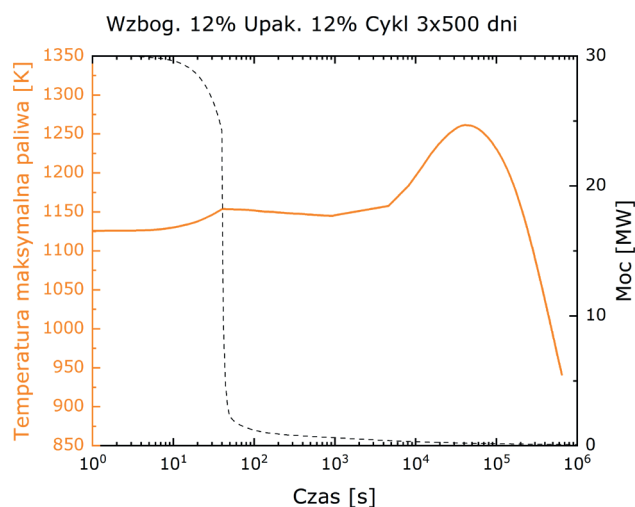
Rys. 6. Rozkład maksymalnej temperatury osiąganey w rdzeniu V2 podczas PLOFC, EOC, wzbogacenie o 12%
