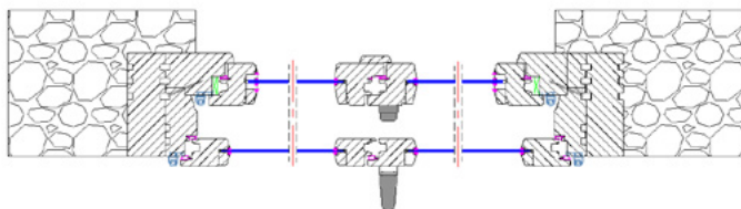
Rys. 1. Przekrój poziomy dotychczasowego rozwiązania
