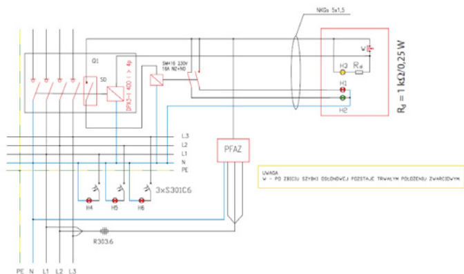
Rys. 3. Schemat ideowy zasilania i sterowania PWP z cewką wzrostową (WW) z kontrolą ciągłości obwodu
