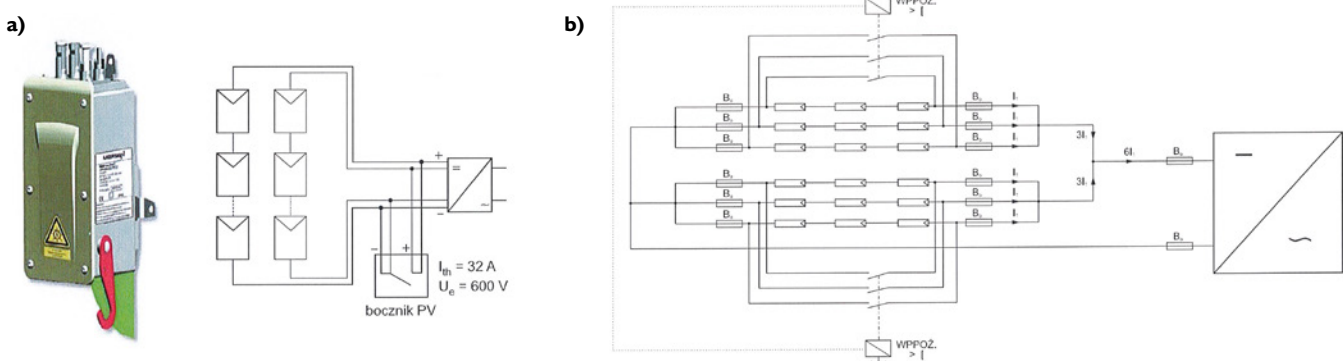
Rys. 7. Przykład wyłączenia pożarowego generatora PV: a) prostego, b) złożonego
