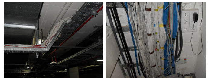
Fot. 3. Przepelnione koryta kablowe, błędne prowadzenie kabli teletechnicznych z innymi kablami
