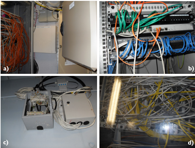
Fot. 1. Błędna realizacja punktu styku: a) punkt styku w pomieszczeniu elektrycznym (błąd projektowy); b) szafa w głównym punkcie styku w pomieszczeniu elektrycznym (błąd projektowy); c) punkt styku na drodze przejazdu w garażu podziemnym (błąd projektowy); d) chaos w głównej szafie krosowej w punkcie styku (błąd wykonawczy).
